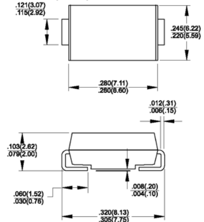
DO-214AB (SMC)
