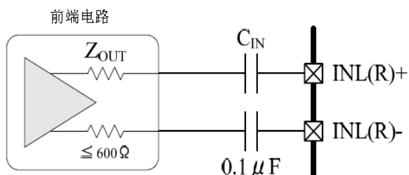
图2. 差分输入
