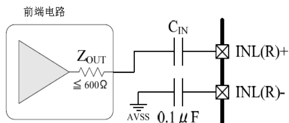
图3. 单端输入
