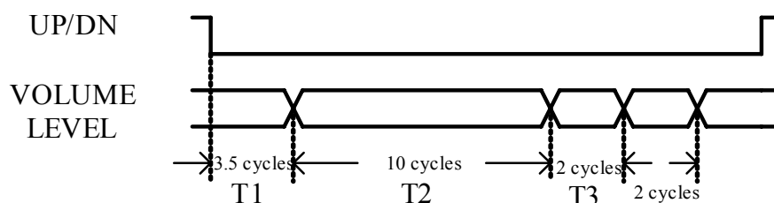
图1. 音量控制时序图
