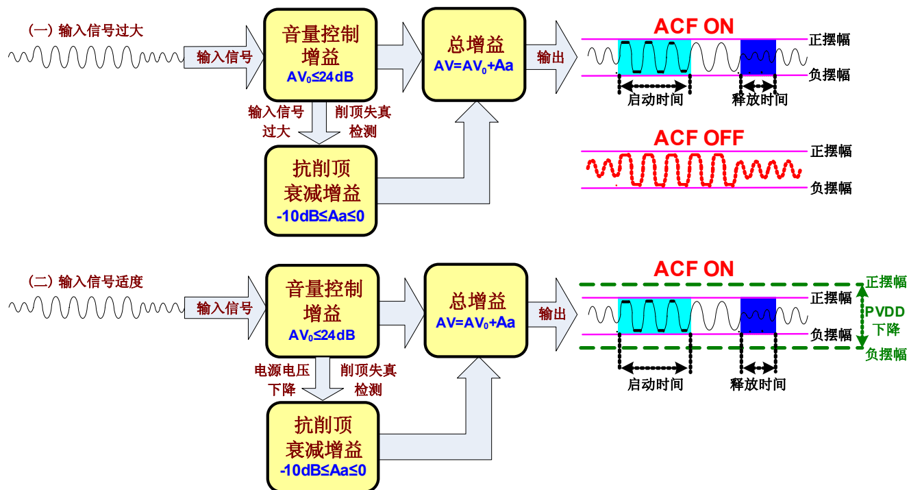
图5. 抗削顶失真功能(ACF)的原理框图
