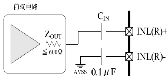
图2. 单端输入
